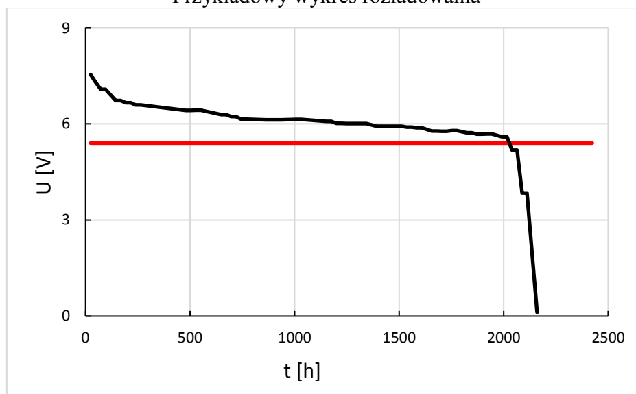
Przykładowy wykres rozładowania
