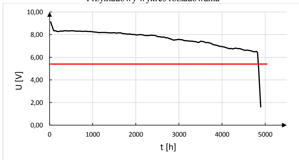
Przykładowy wykres rozładowania
