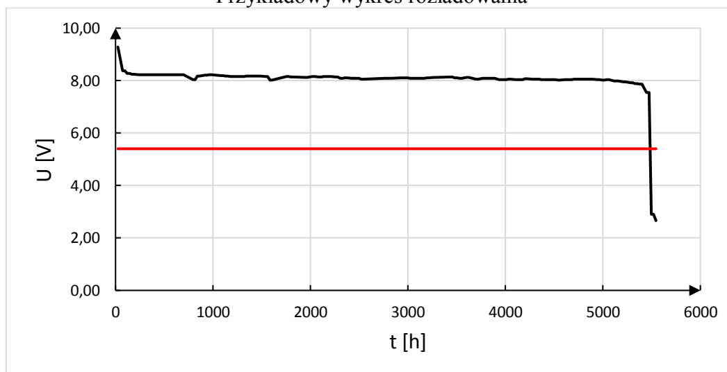
Przykładowy wykres rozładowania
